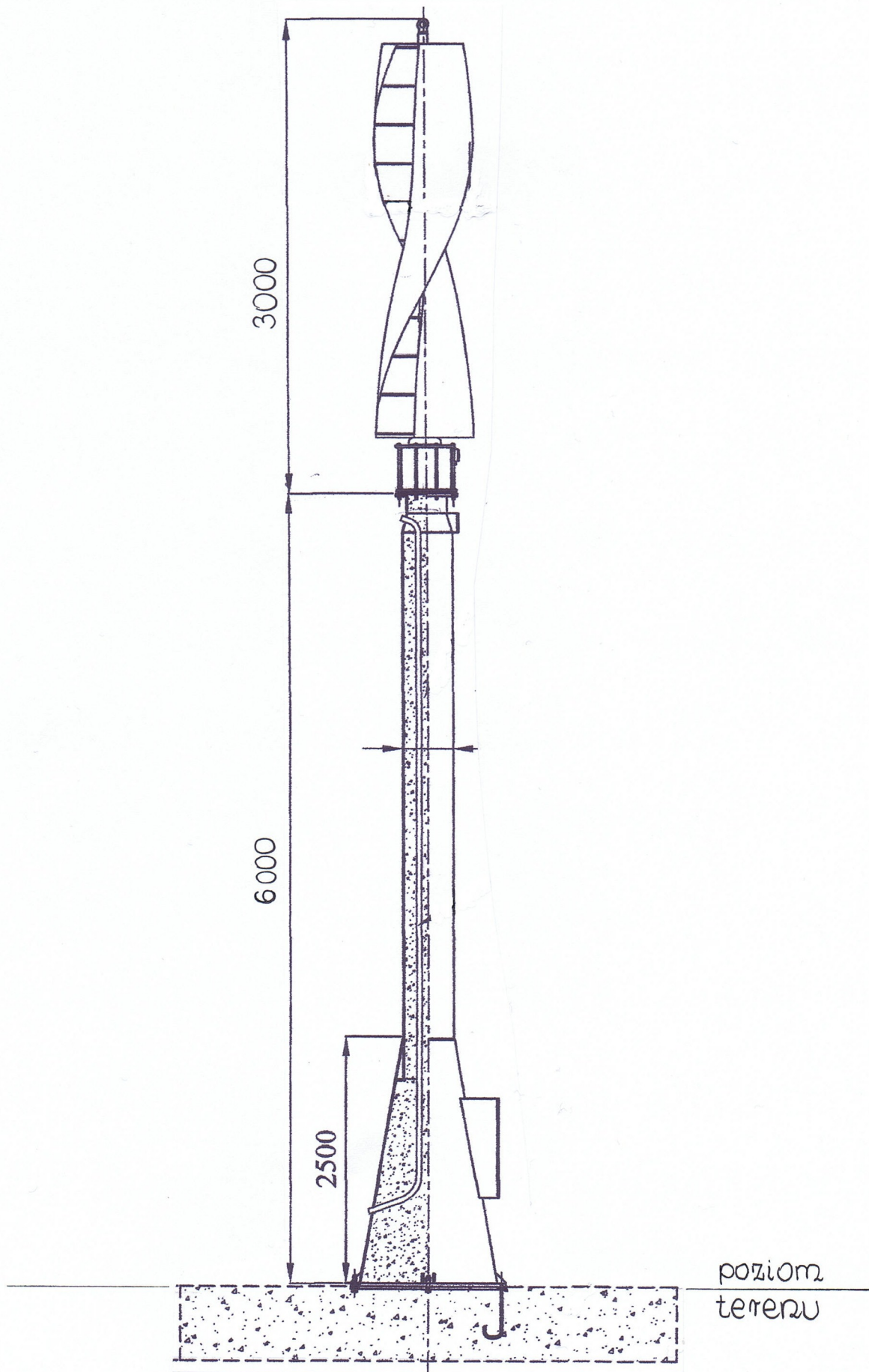
Rys. nr 2 - przykładowy schemat posadowienia turbiny wiatrowej
